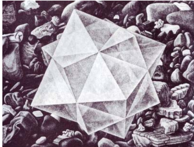
FIG 2 - Il cristallo
