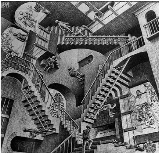
FIG 3 - Relatività
